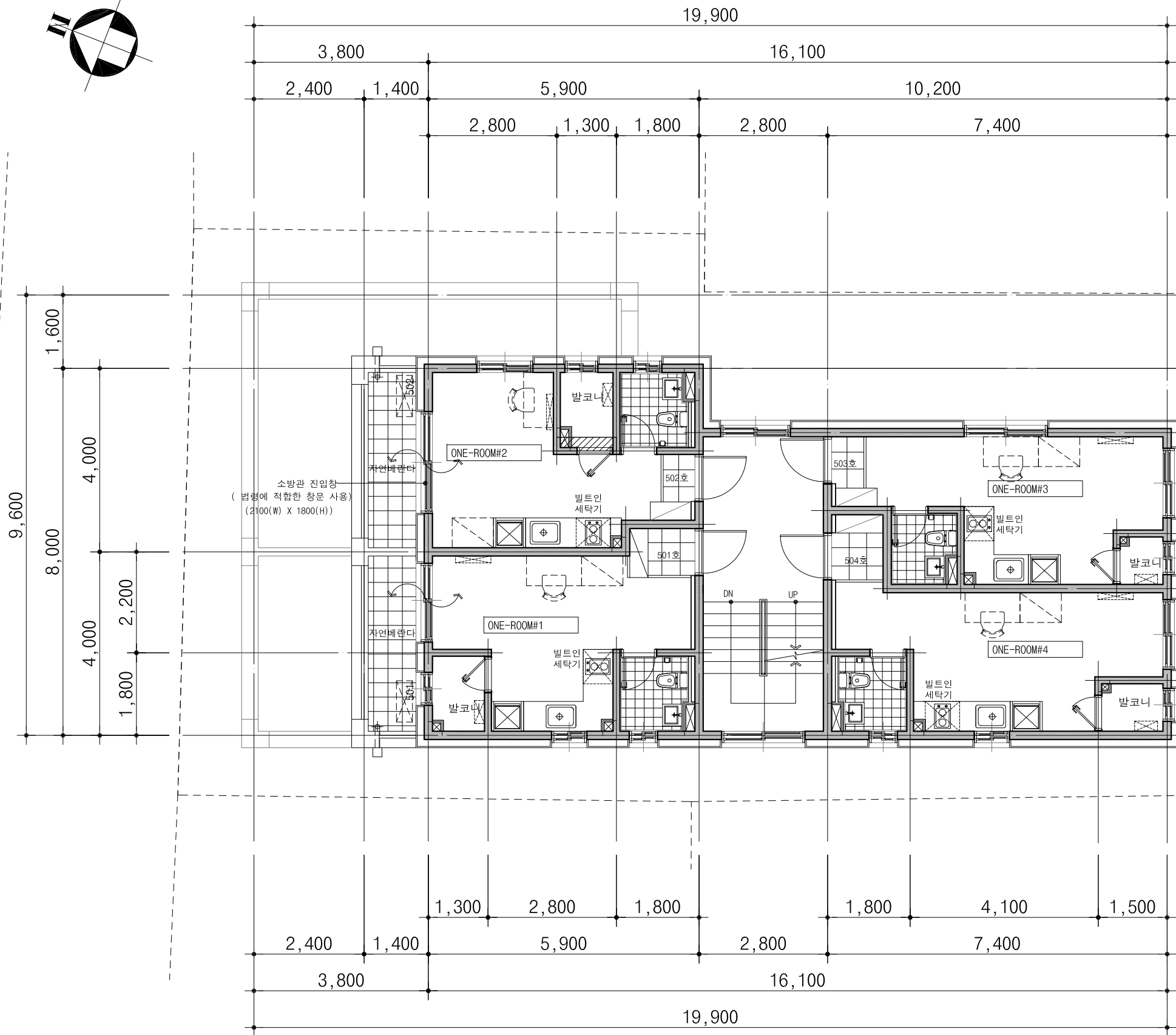
5 층 평 면 도 SCALE: 1/100
