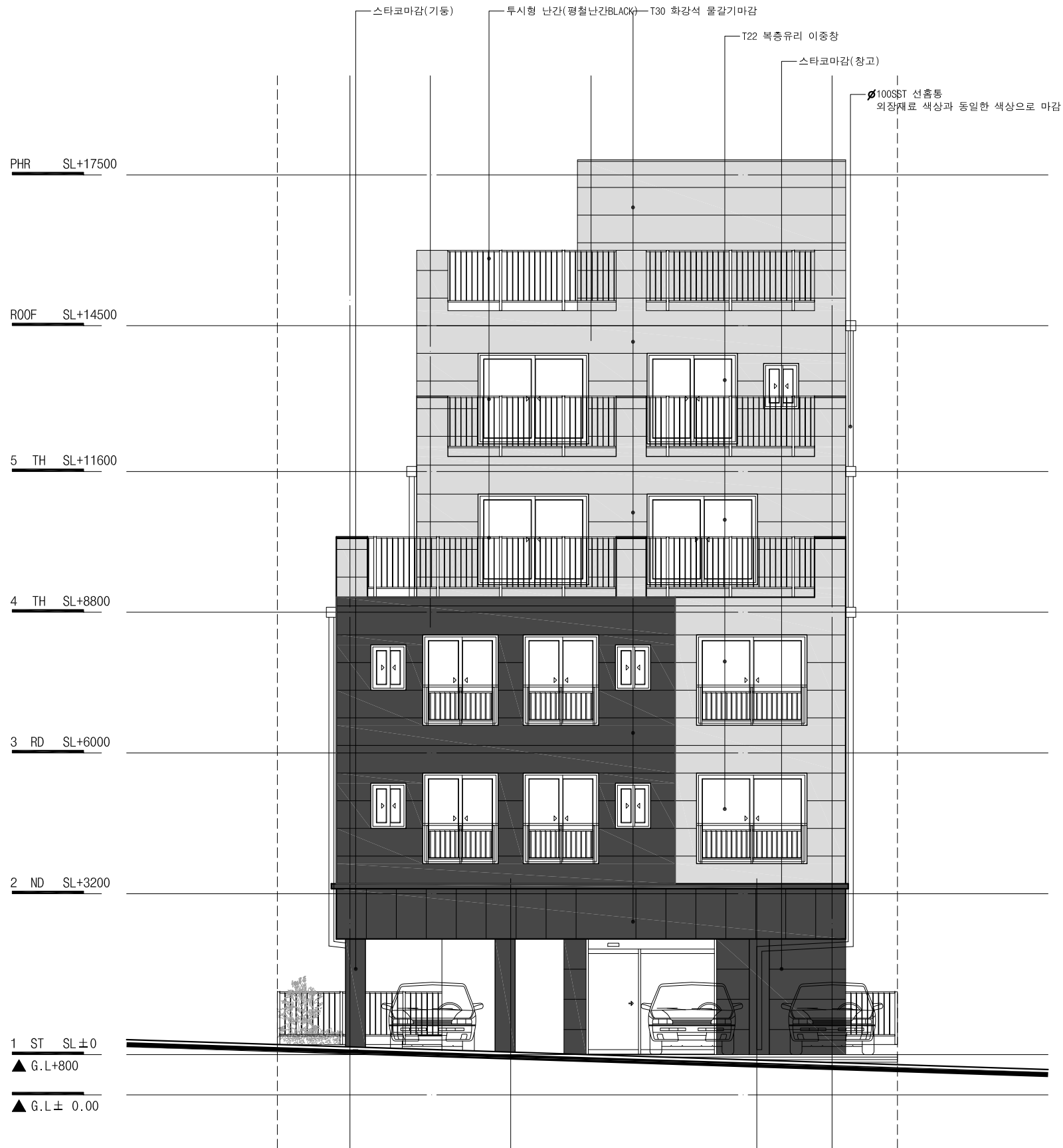
정 면 도 SCALE: 1/100
