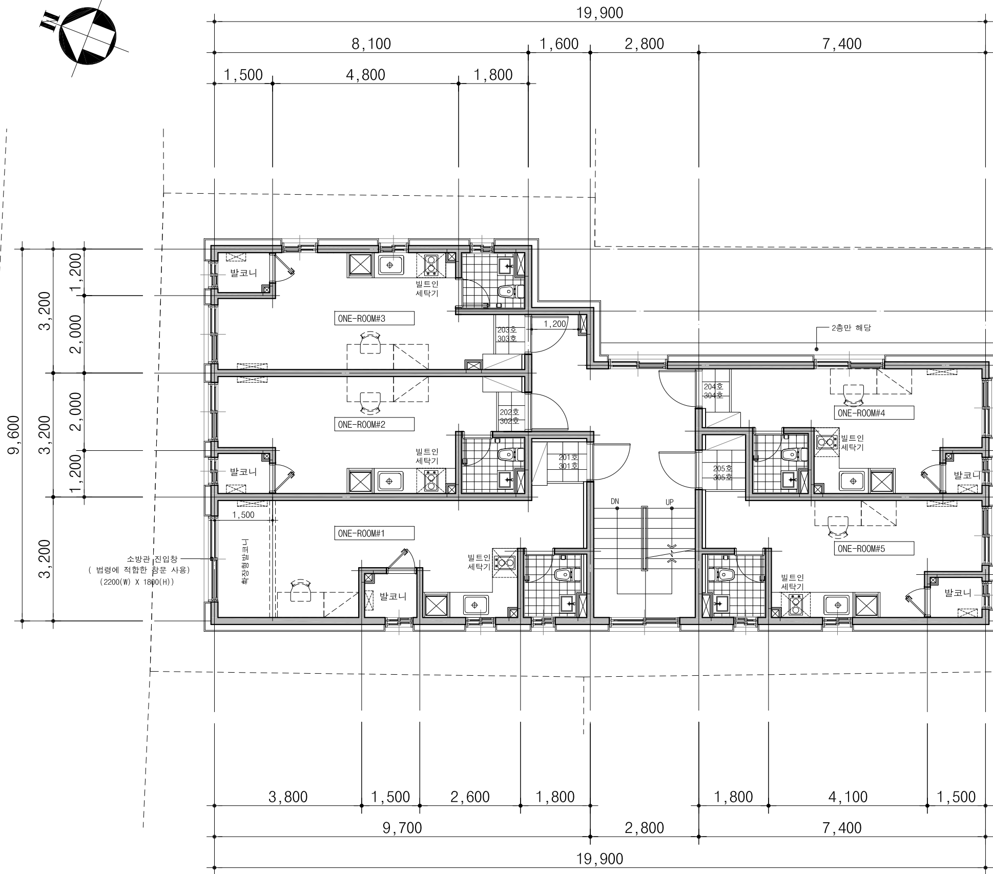
2 ~ 3 층 평 면 도 SCALE: 1/100
