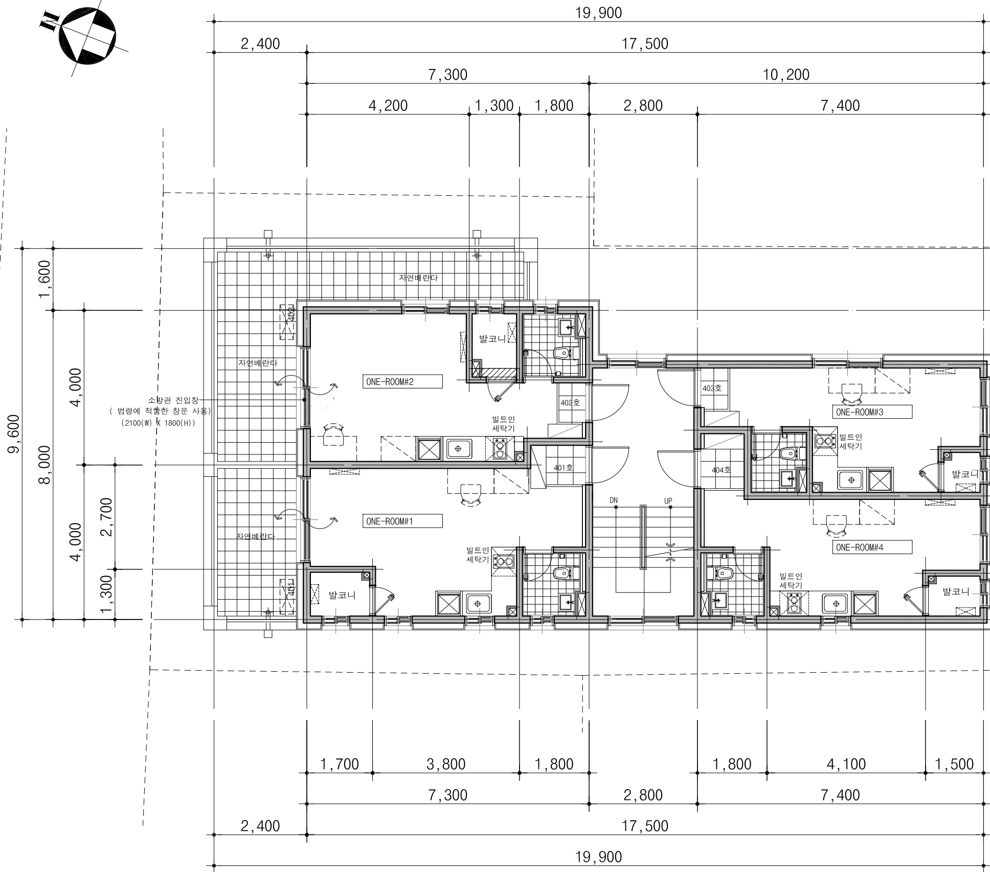
4 층 평 면 도 SCALE: 1/100
